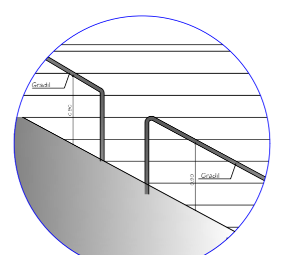
Detalhe Gradil: Sem Escala
